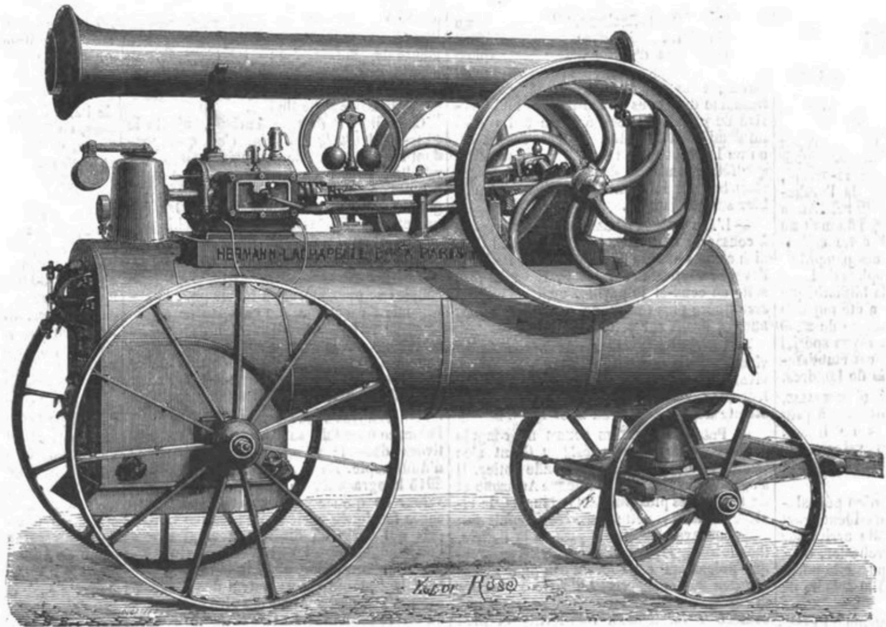
EXPOSITION DE MACHINES AGRICOLES AU PALAIS DE L'INDUSTRIE. — MACHINE A VAPEUR HORIZONTALE LOCOMOBILE MONTÉE SUR TRAIN DE ROUES, construite par J. HERMANN-LACHAPELLE, ingénieur-mécanicien, 144, faubourg Poissonnière, Paris.
